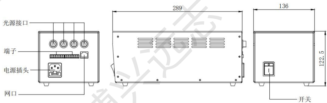
图 1-1 高精度数字电源机械尺寸图
